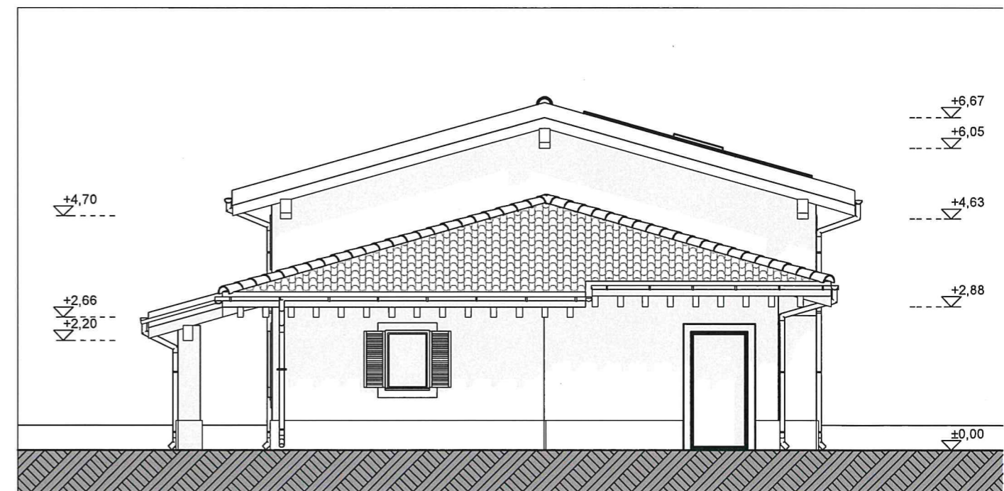
PROSPETTO NORD-OVEST
