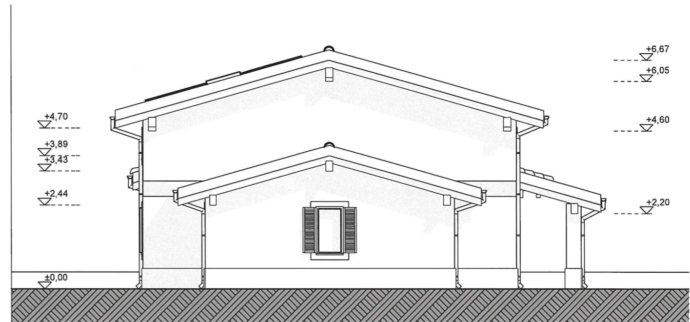
PROSPETTO NORD-OVEST
